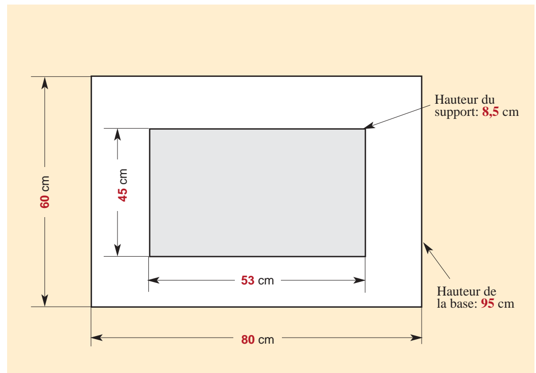
Croquis des supports en bois de la statue de la “ Vierge de l’Espérance ”.
