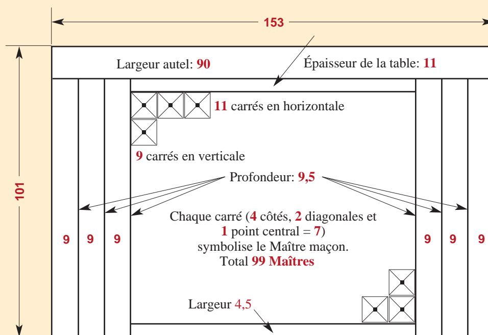
Croquis de la vue frontale de l'autel de la cryptte avec les dimensions en centimètres.
